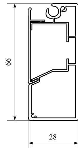
D apakšēja slīde
