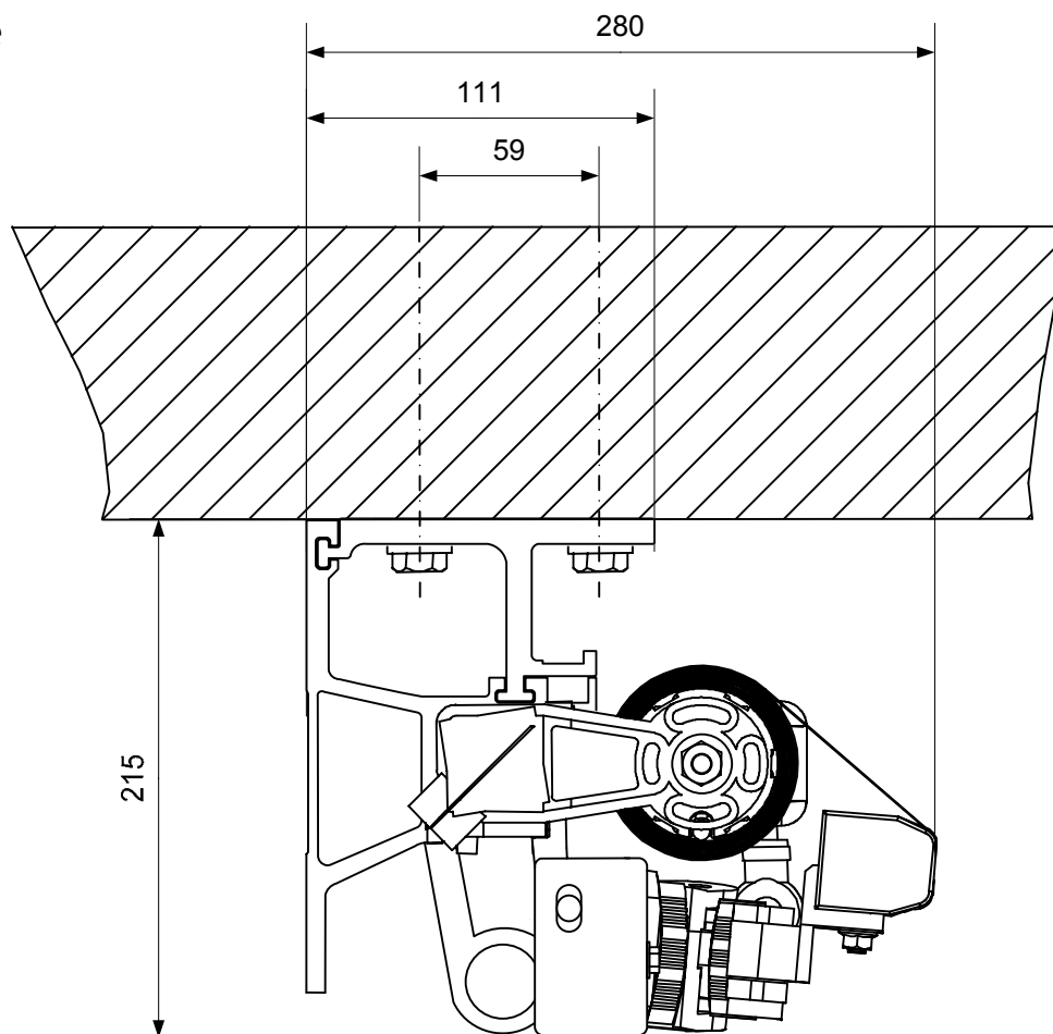
Montāža griestu plaknē
