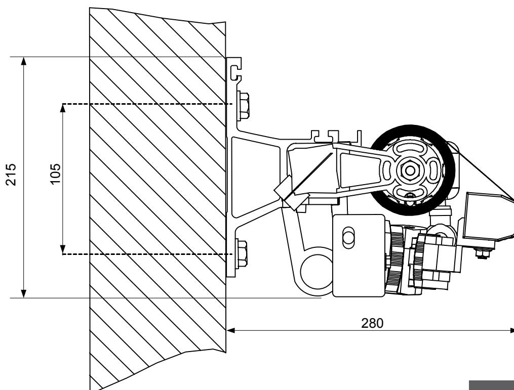
Montāža sienas plaknē
